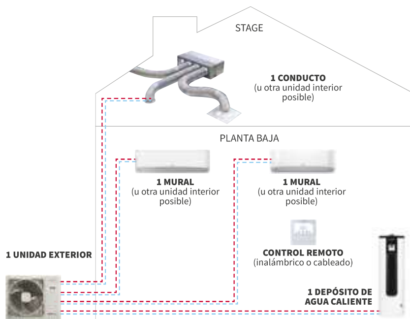
Ejemplo instalación
